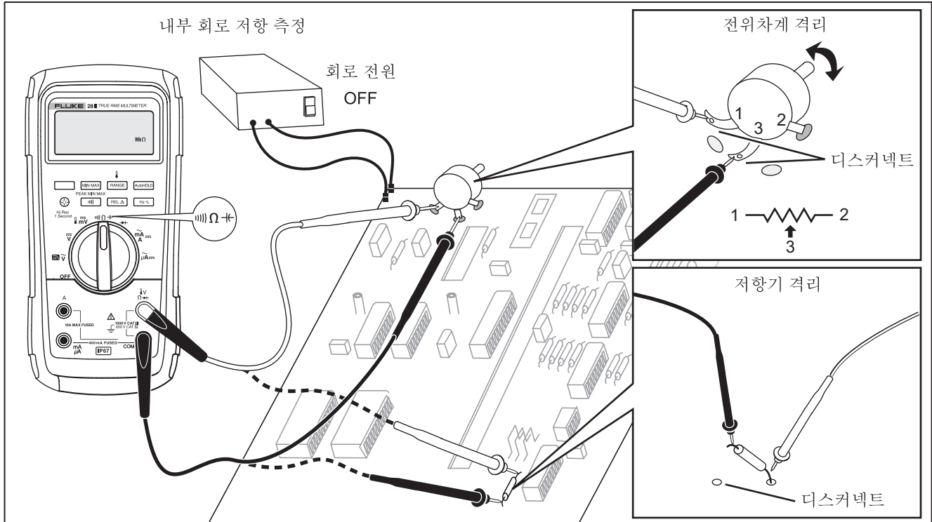
그림 5. 저항 측정
